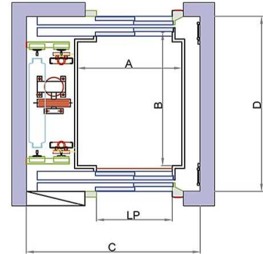
Entradas opostas (2)
