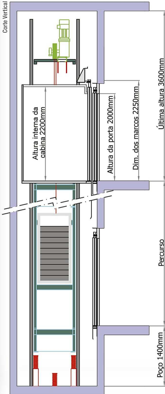
Planta da Caixa - Abertura Lateral
