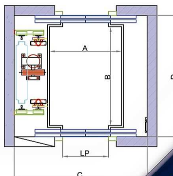
Entradas opostas (2)
