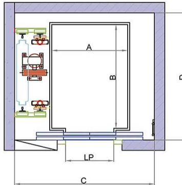
Entrada unilateral (1)
